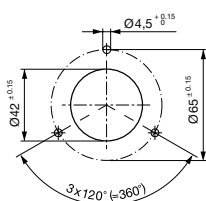
Durchgangsbohrung
