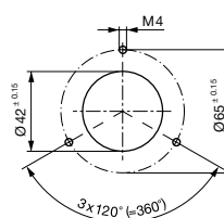
Gewindebohrung
