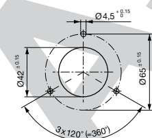
Durchgangsbohrung
