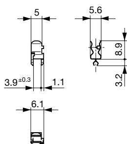
Varianten 2 0751.0110 und 0751.0231
