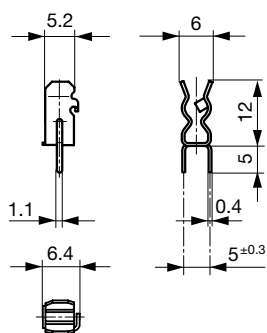
Variante 0751.0052 und 0751.0062
