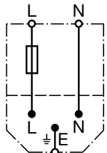
Version ohne Anzeigelampe
