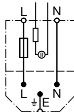
Version mit Anzeigelampe
